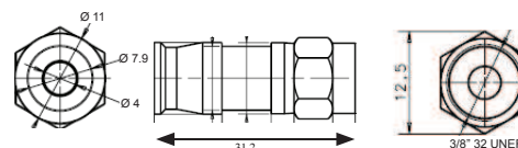
Réf. 4105
