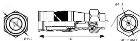
Réf. 4106
